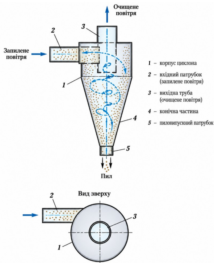
Рисунок 4.1. Схема циклону:
