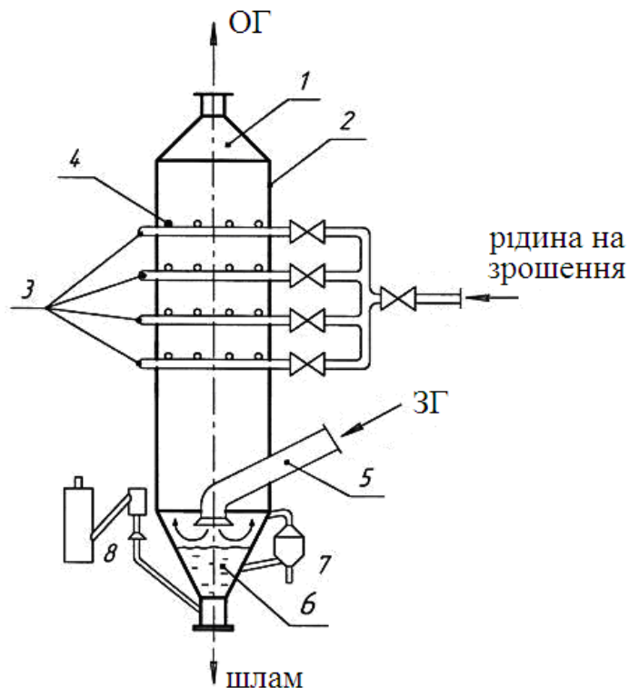
Рисунок 5.2 – Конструктивна схема багатоярусного форсункового скрубера
