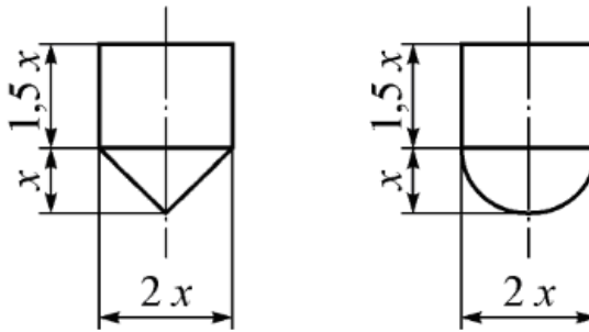
Рисунок 2.9 – Перетини лотків (жолобів) різних конструкцій
