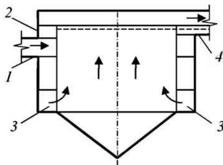
Рис. 1.3 – Вертикальний пісковловлювач з обертовим рухом потоку рідини
