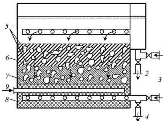
Рисунок 2.5 – Схема каркасно-засипного зернистого фільтра
