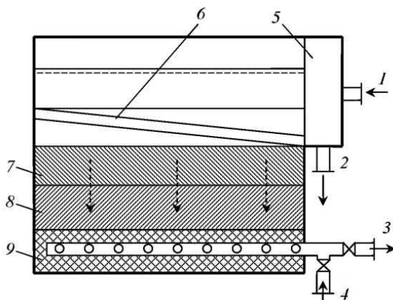
Рисунок 2.3 – Схема двошарового зернистого фільтра
