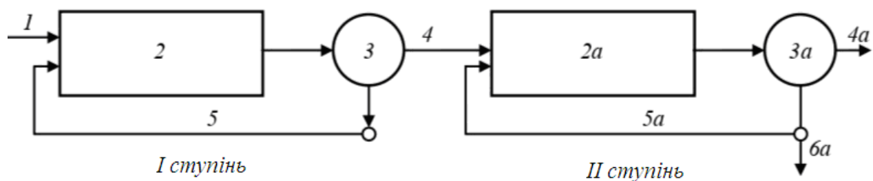
Рисунок 3.5 – Двоступінчаста схема очищення стічних вод в аеротенках без регенерації
