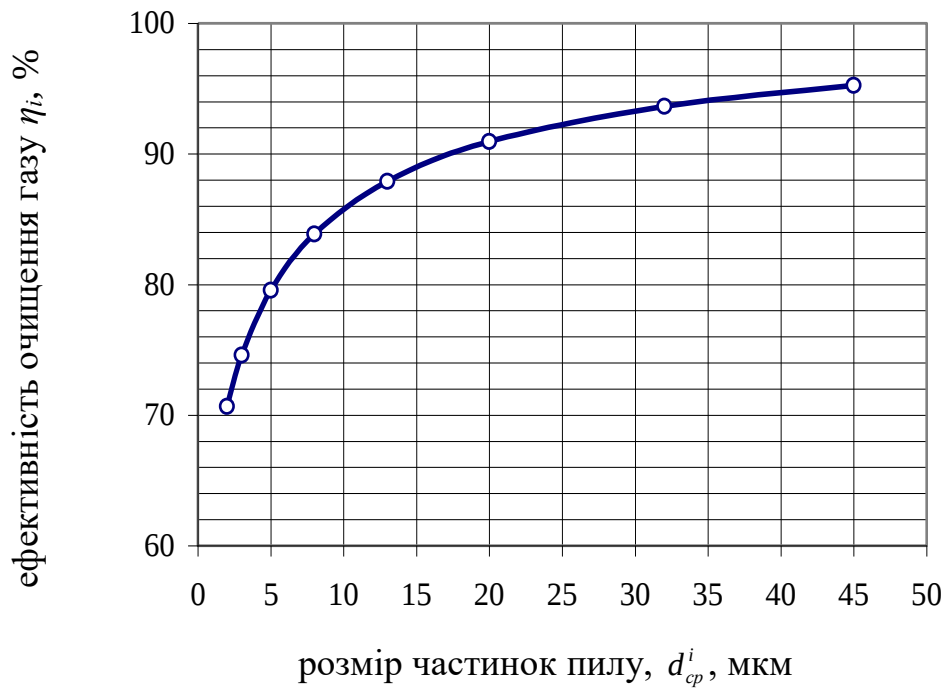
Графік залежності ефективності очищення газу в батарейному циклоні типу БЦ-2 від фракційного складу пилу
