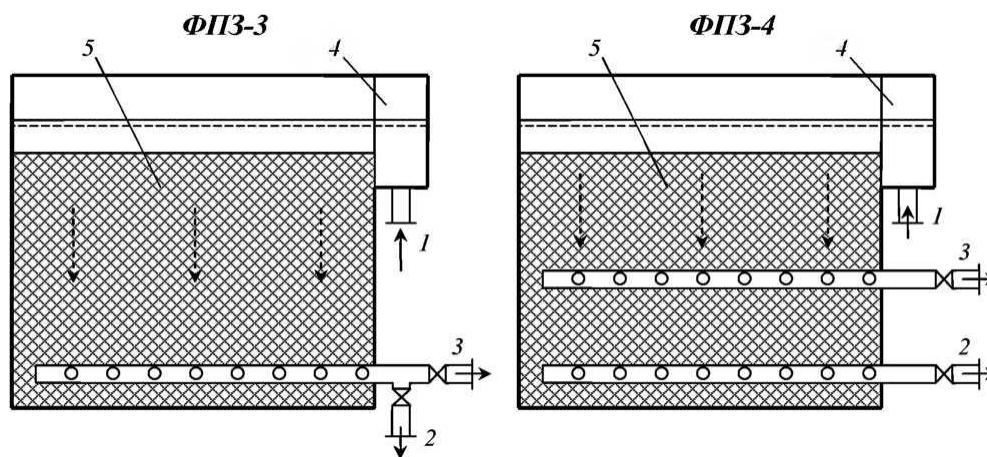
Рисунок 2.6 – Схема фільтрів з плаваючим завантаженням із спіненого полістиролу
