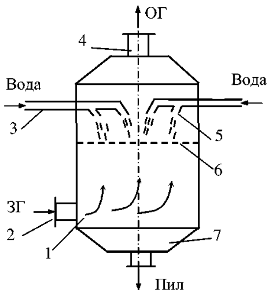
Рисунок 5.1 – Конструктивна схема форсунокового протиструминного скрубера
