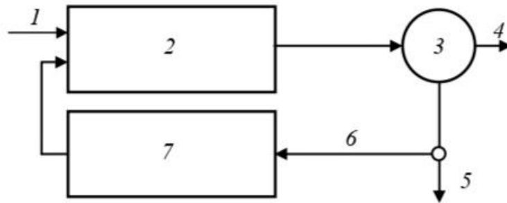
Рисунок 3.4 – Одноступінчаста схема очистки в аеротенках з регенерацією
