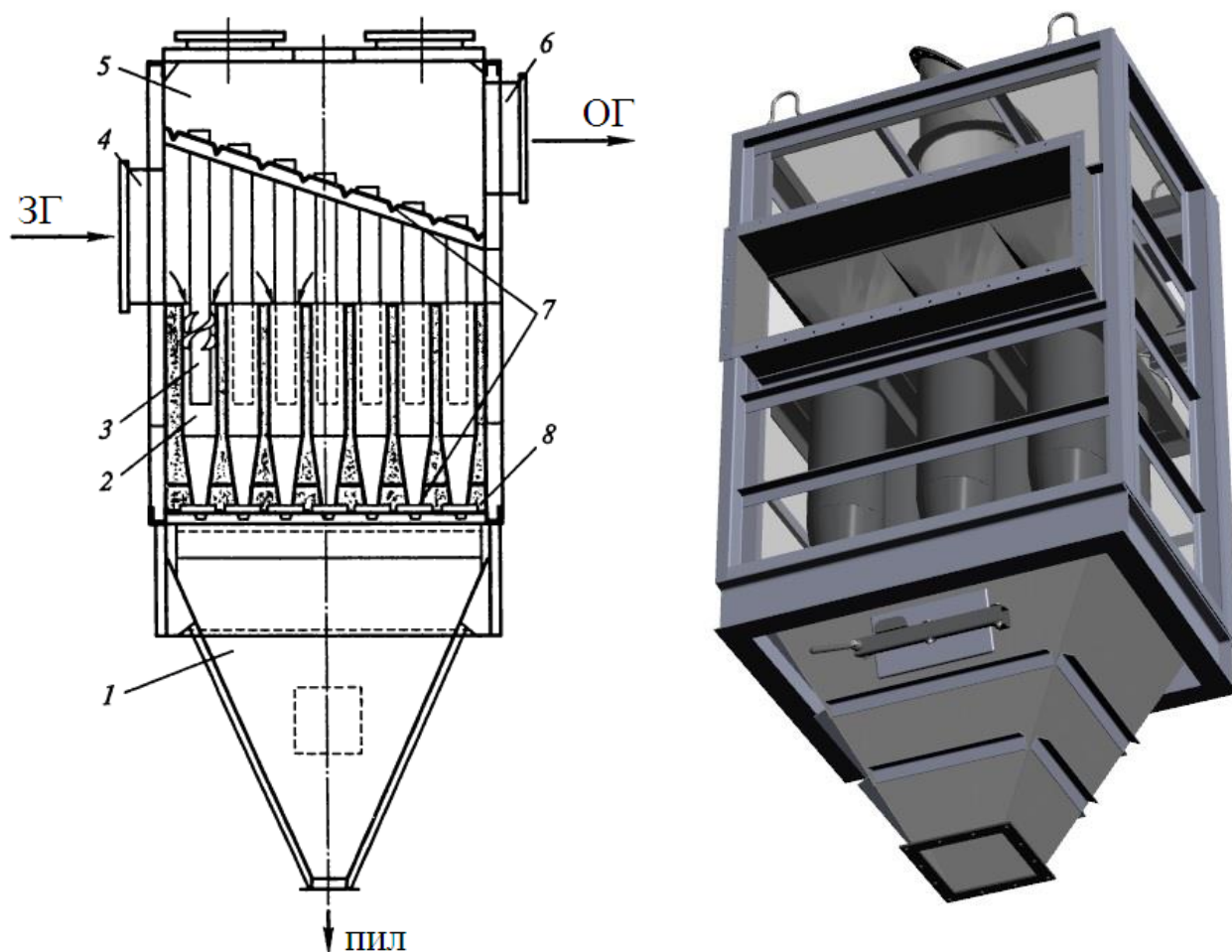
Рисунок 4.1 – Конструктивна схема батарейного циклону
