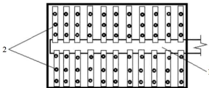
Рисунок 2.8 – Дренажна (розподільча) система одношарового фільтра з дрібнозернистим піщаним завантаженням
