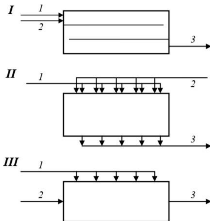
Рисунок 3.6 – Типи аеротенків
